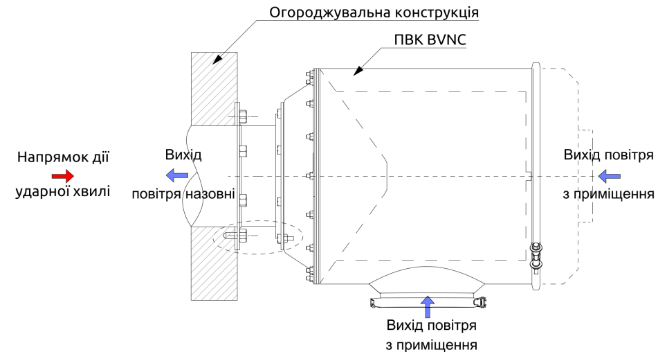
Схема пристрою ПВК BVNC (Нормально зачинені клапани BVNC можуть бути встановлені лише на витяжних або рециркуляційних отворах, фланцем в бік ударної хвилі)
