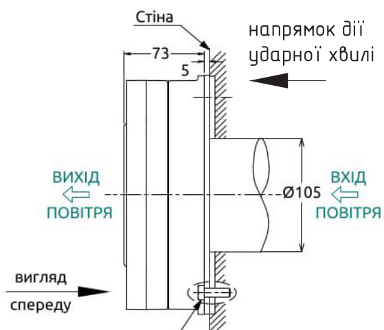
ВИГЛЯД ЗБОКУ
