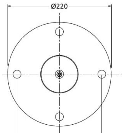
ВИГЛЯД СПЕРЕДУ
