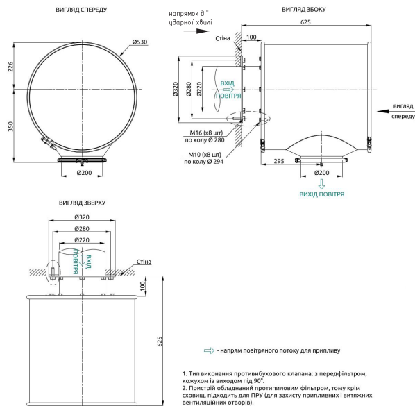
Габаритні та присднувальні розміри BVNO 1800 8Z
