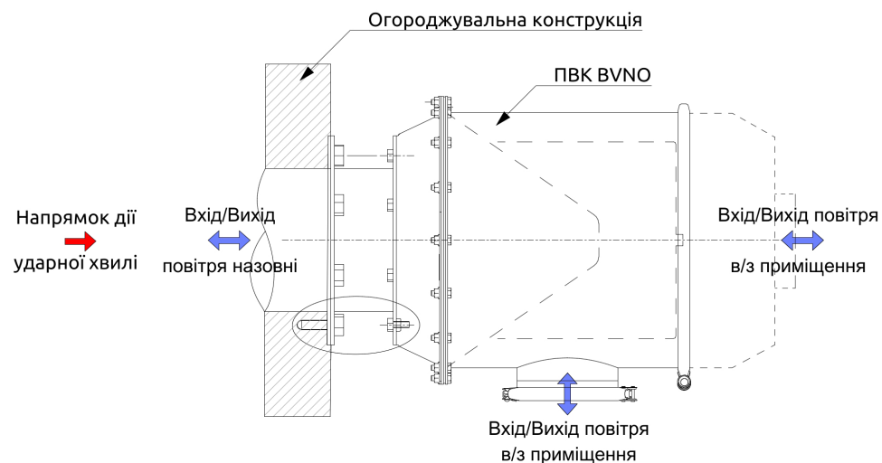
Схема пристрою ПВК BVNO
