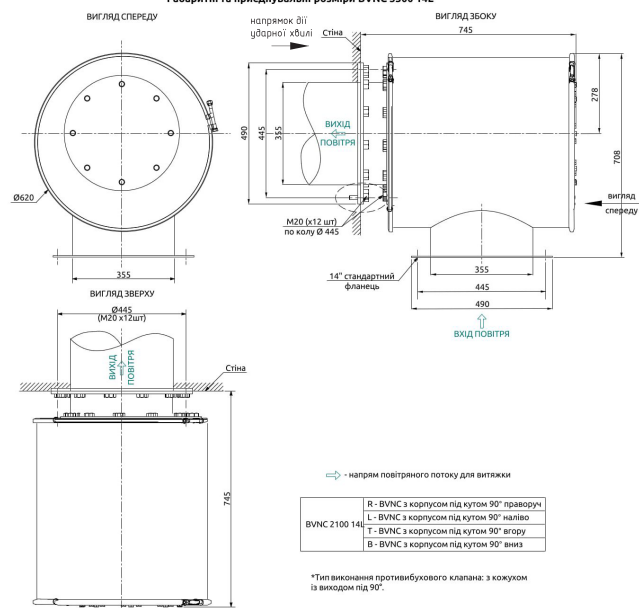
Габаритні та присудувальні розміри BVNC 3300 14Z
