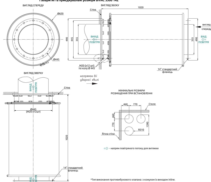
Габаритні та присудувальні розміри BVNC 3300 14Z
