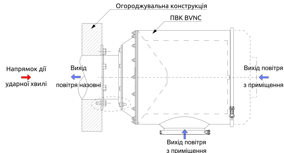
Схема пристрою ПВК BVNC
