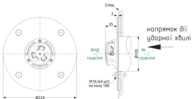
Габаритні та приєднувальні розміри BVNC 40 4Y
